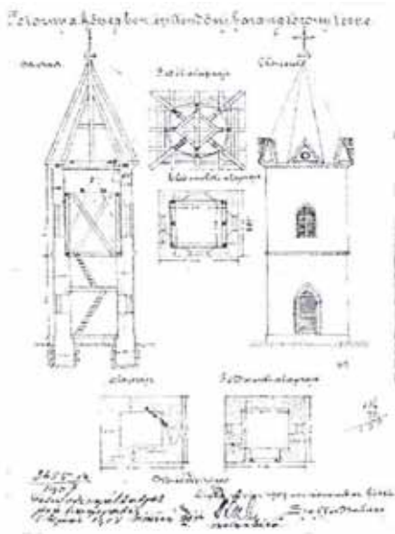
Plán na stavebné projekty pôvodnej zvonice
